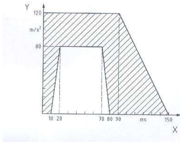
شکل ۶- حرکت شتابی
