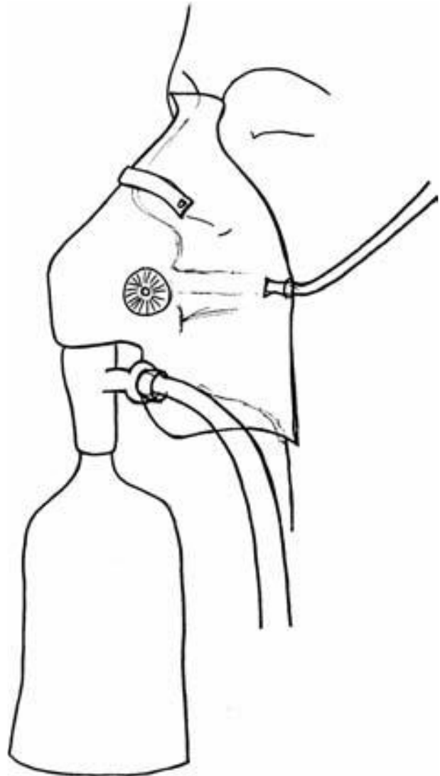
شکل ۵-۹: ماسک فاقد ویژگی تنفس مجدد (همراه با کیسه منبع ذخیره)
